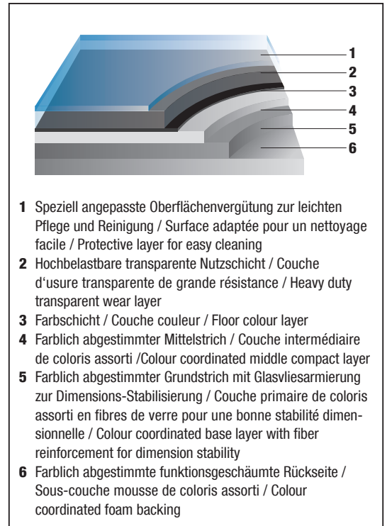
Bodenaufbau / Construction du tapis / Layer Structure
